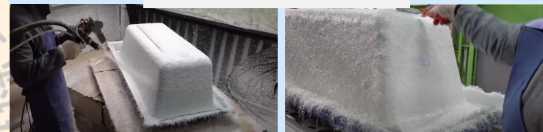
玻璃纖維強化塑膠(FRP/塑鋼)生產過程
