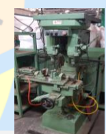
傳統立式 雙軸加工機
